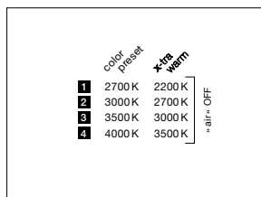
4. Mögliche, einstellbare Farbtemperaturen entsprechend gewählter Konfiguration (color preset oder »x-tra warm«). touchless control und Occhio air sind deaktiviert, Phasenabschnittdimmung möglich.
